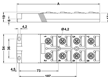
SACB-...HPUR, dubbelkontakt
