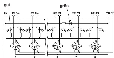
Plintkonfiguration: SACB-..., dubbelkontakt. (för pnp-sensorer / aktorer) Ledaranslutning, se tabell.
